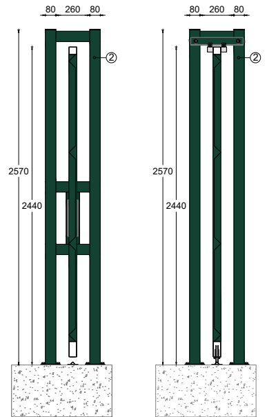
CORTE A
