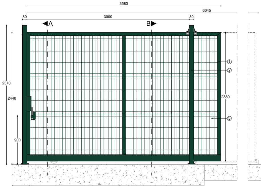
ALÇADO
