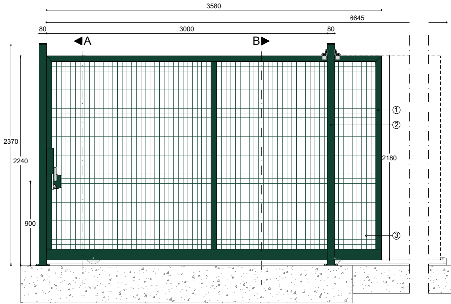
ALÇADO
