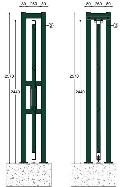
CORTE A
